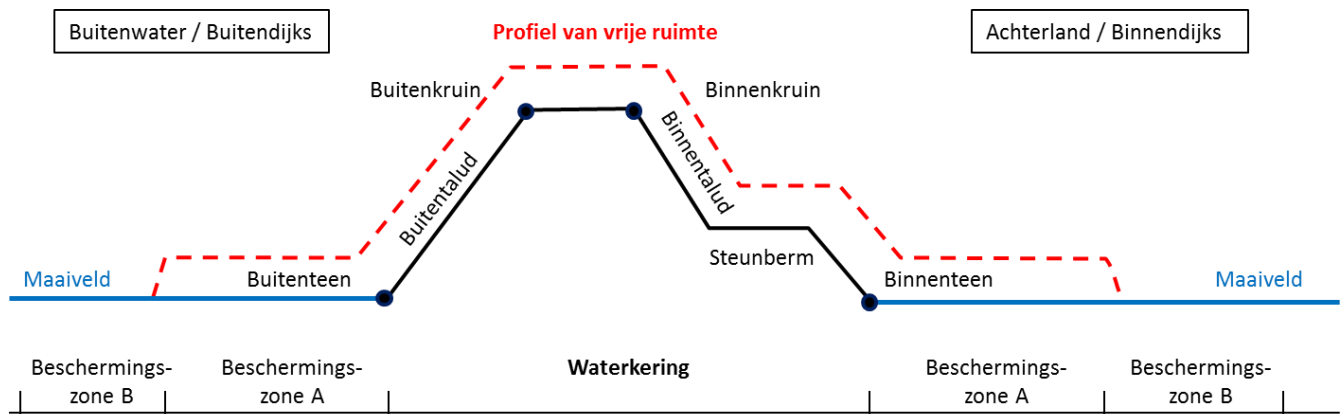
Figuur 15.2: Principe van leggerprofiel en bijbehorende zones en profiel van vrije ruimte
